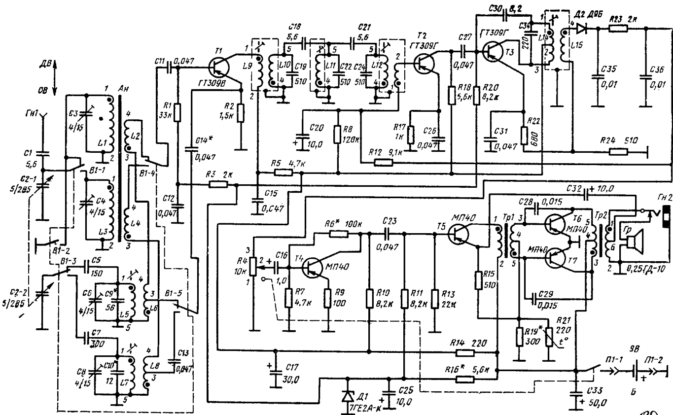
Принципиальная электрическая схема радиоприемника «Кварц-407»
